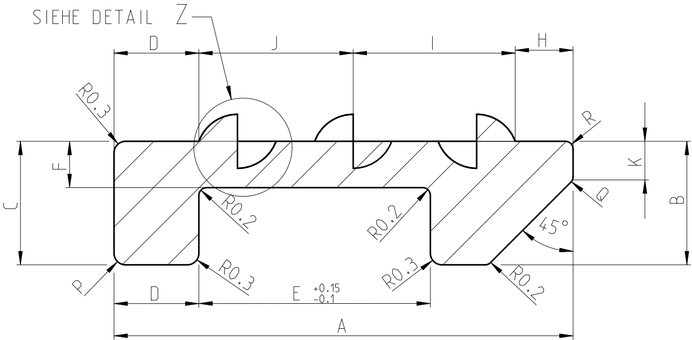
Profilquerschnitt 10:1
